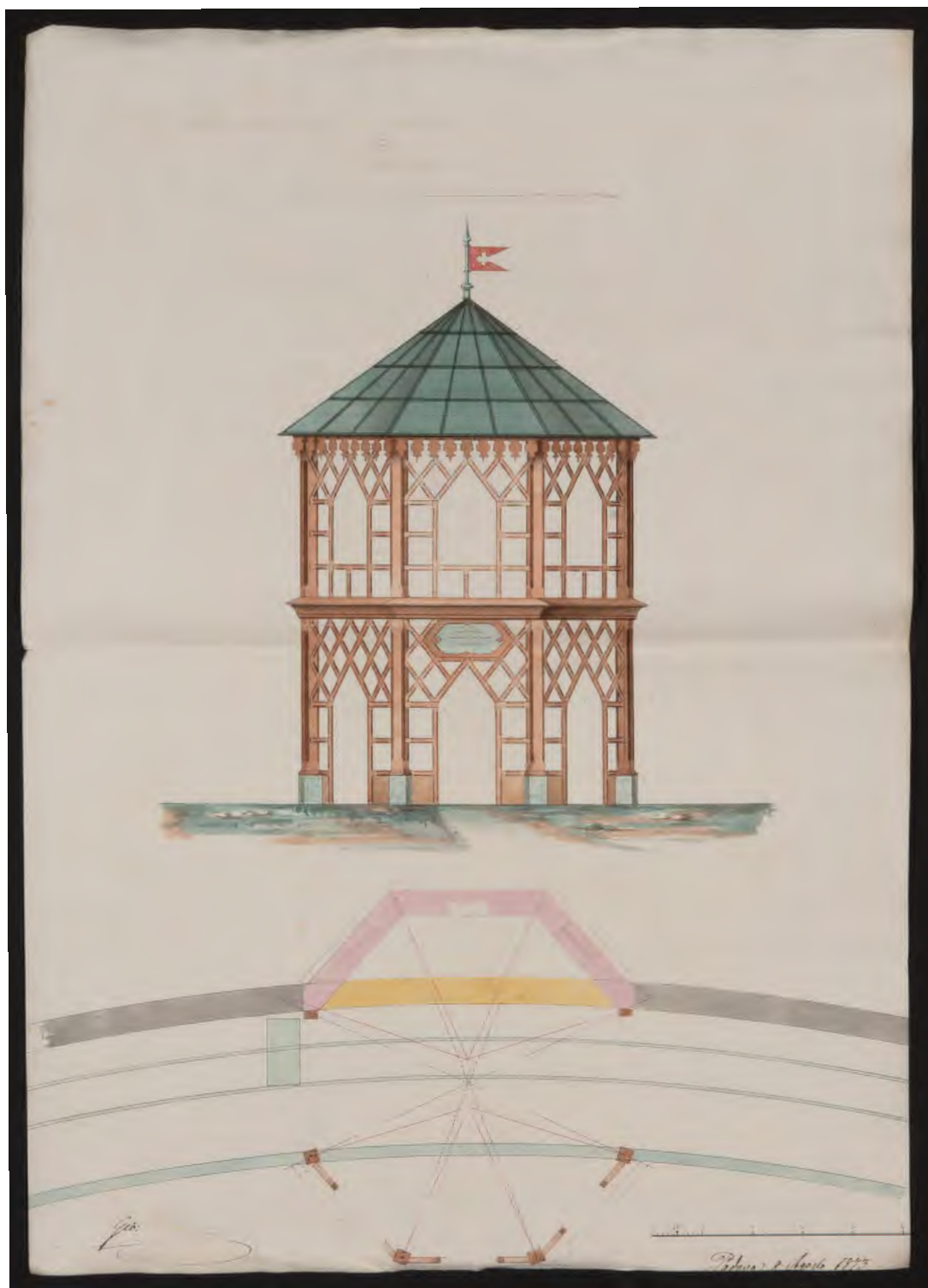
FIG. 8 – Tipi della nuova serra pella palma di Goethe che servirono di base al primitivo Fabbisogno di spesa. Disegno acquerellato policromo su carta pesante, relativo al progetto per la nuova costruzione della serra della palma di Goethe, 8 agosto 1873. Biblioteca storica di medicina e botanica Vincenzo Pinali e Giovanni Marsili, 12/4 – Ar.B.6.B (Phaidra: < https://hdl.handle.net/11168/11.456044 >).
